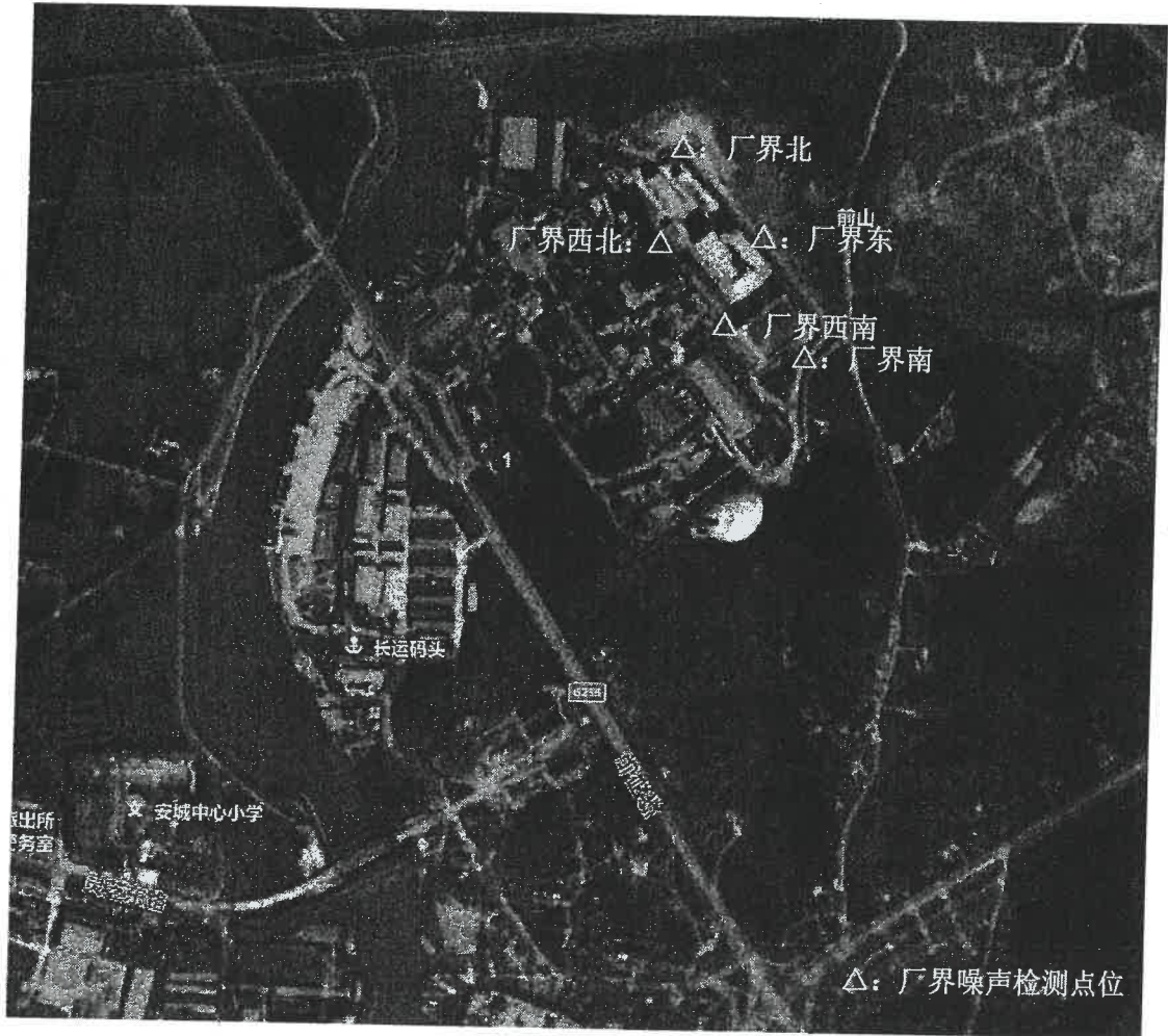
安吉纳海环境有限公司噪声检测点位示意图
